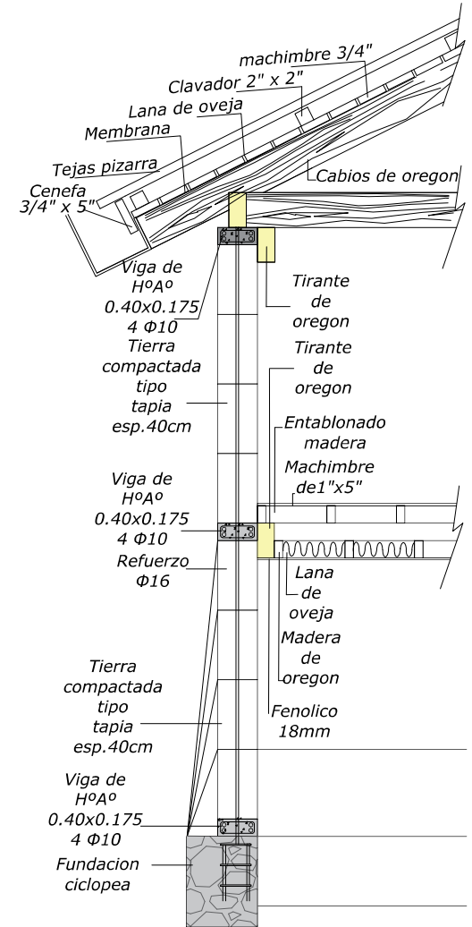
CORTE CONSTRUCTIVO 1:25
