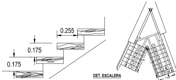
DET. ESCALERA
