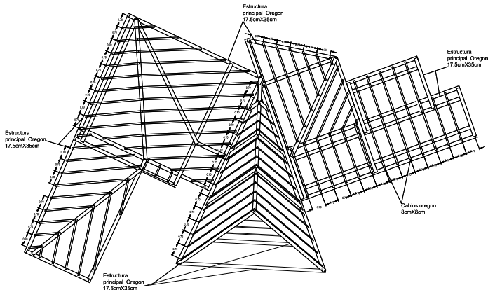
PLANTA ESTRUCTURA DE TECHOS 1:100
